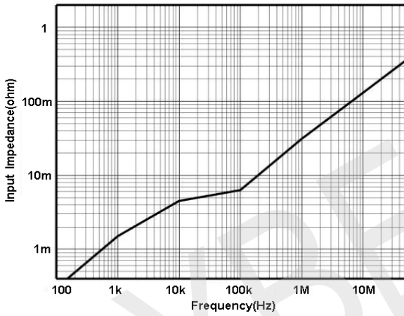
图 6 HCP8050 输入阻抗 VS 频率曲线
